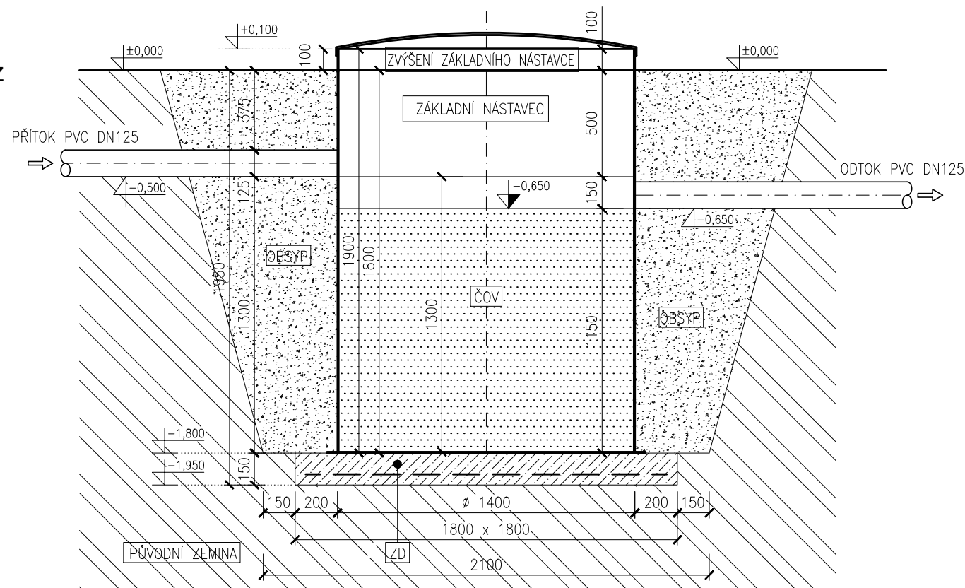
Řez
